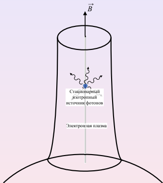
Аккреционная колонка
